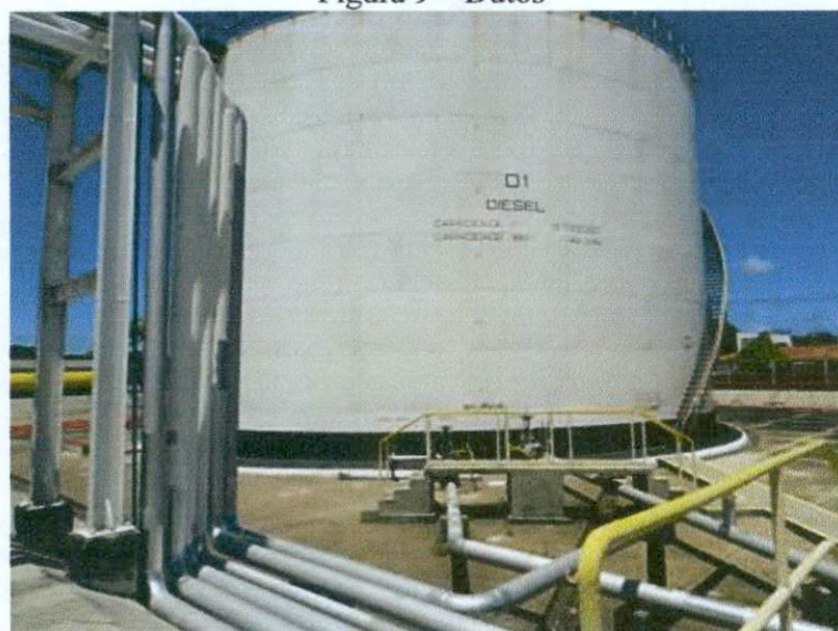
Figura 9 – Dutos
